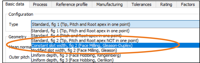
Figure 7. Selecting «constant slot width» type or «modified slot width» type
