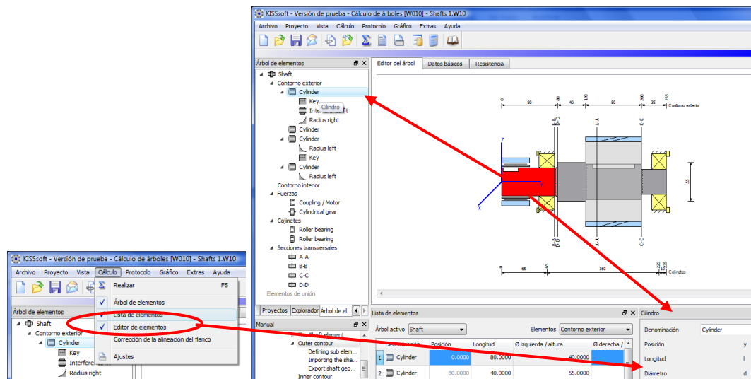
Figura 2.4 Diálogo para visualizar el editor de elementos.
