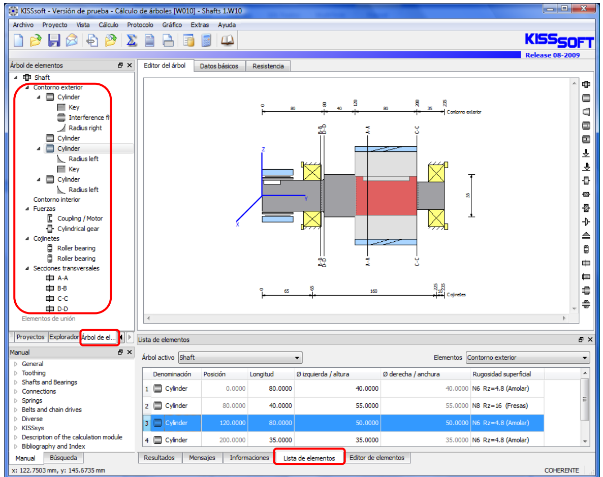
Figura 2.1 Los cinco elementos más importantes para crear un árbol.
