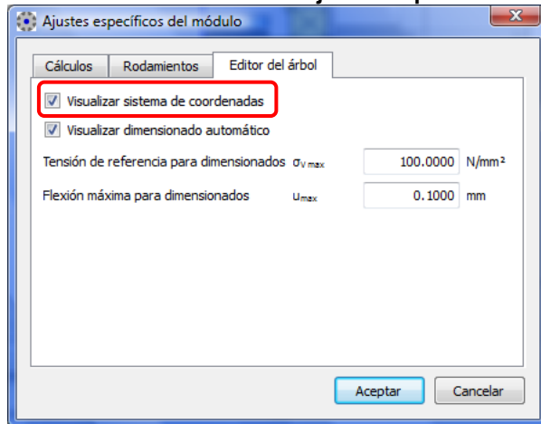
Figura 2.2 Diálogo Editor del árbol en Ajustes específicos del módulo.
