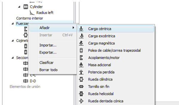
Figura 2.6 Insertar elementos de la máquina.
