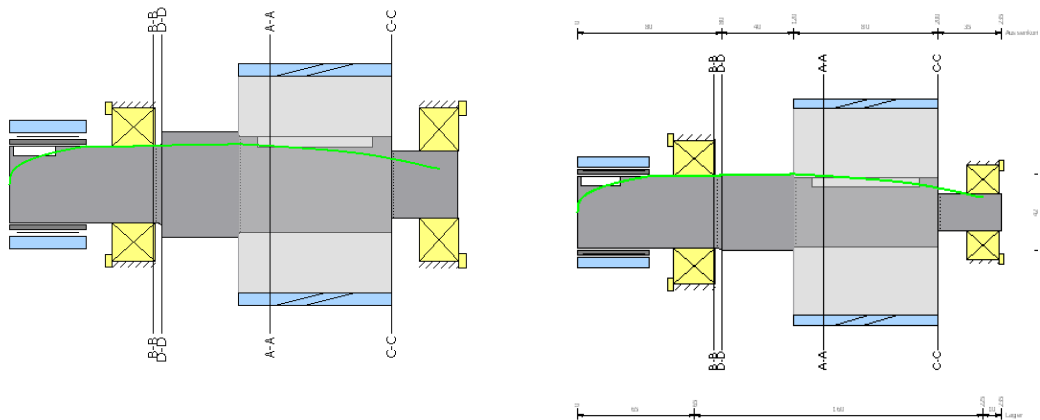
Figura 2.15 Geometría original con propuesta para el recorrido del diámetro (línea verde), a la derecha: Geometría ajustada, llamada del menú «Dimensionar/La resistencia».
