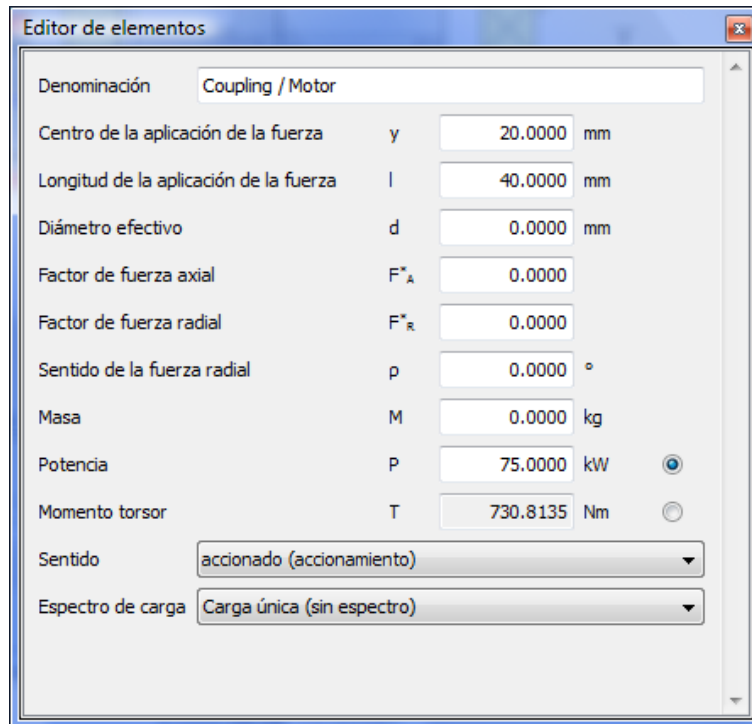
Figura 2.8 Definición del acoplamiento.
