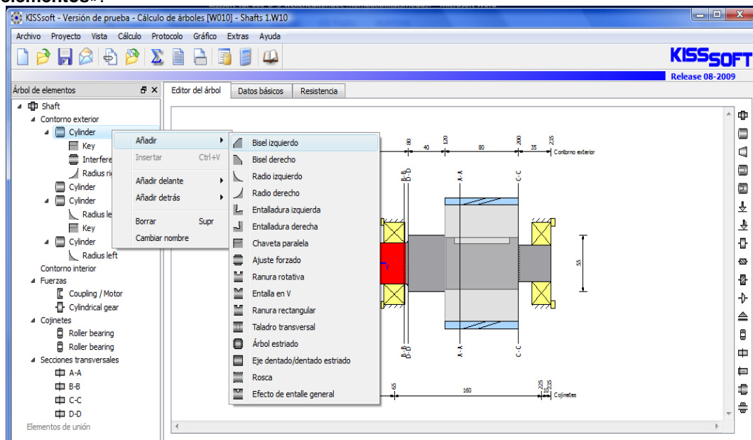
Figura 2.5 Diálogo para definir los elementos auxiliares.
