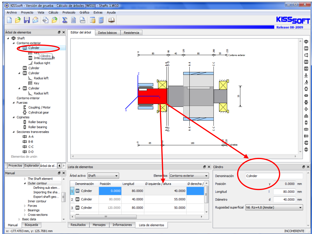
Figura 2.3 Diálogo para la definición de una sección del árbol (cilindro).
