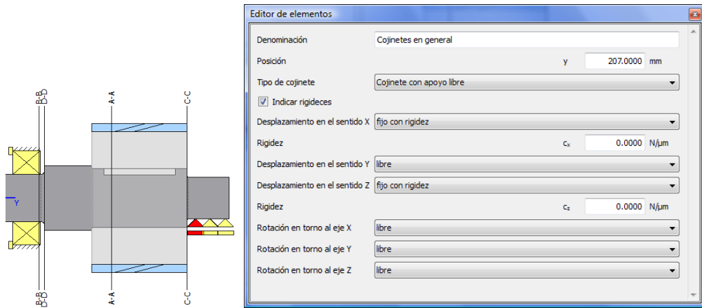
Figura 2.12 Ejemplo para modelar un apoyo en línea con varios cojinetes.
